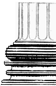
Č. 466. Basis iónská (z chrámu Athénina v Priéné).
